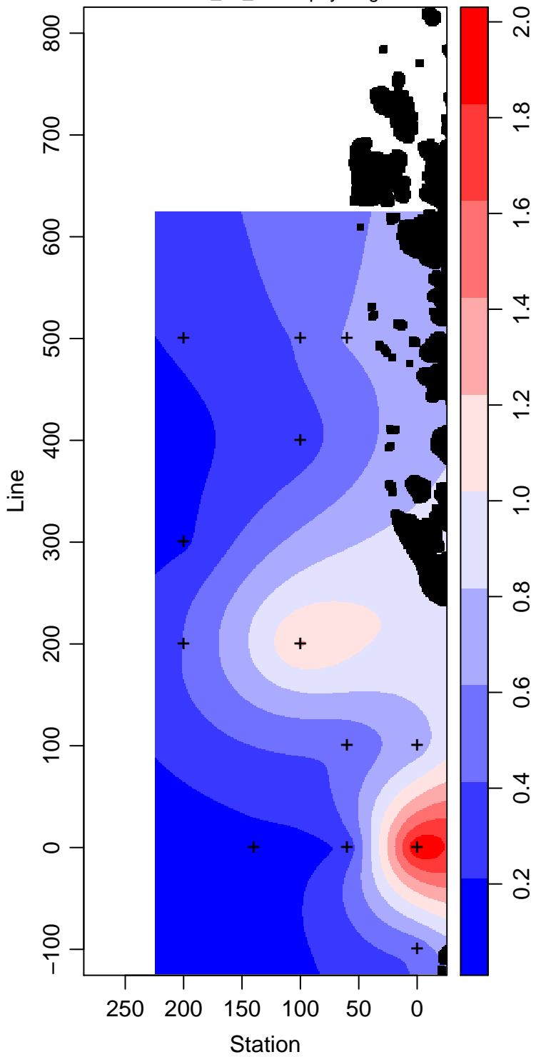
LMG13-01_55_Chlorophyll mg m -3
