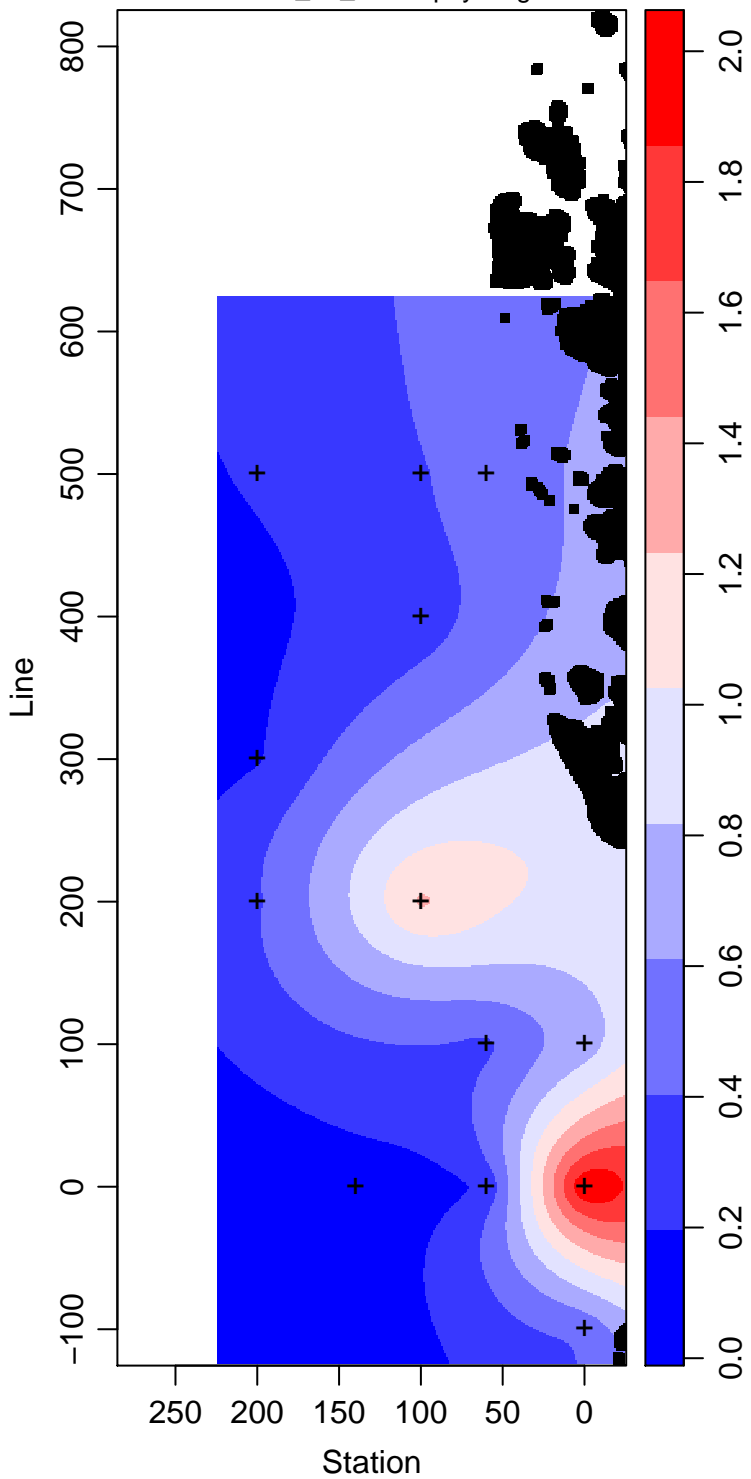
LMG13-01_60_Chlorophyll mg m -3
