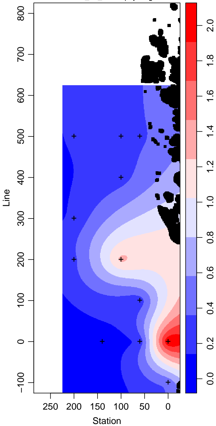
LMG13-01_70_Chlorophyll mg m -3
