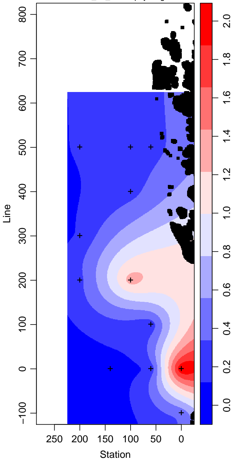
LMG13-01_75_Chlorophyll mg m -3
