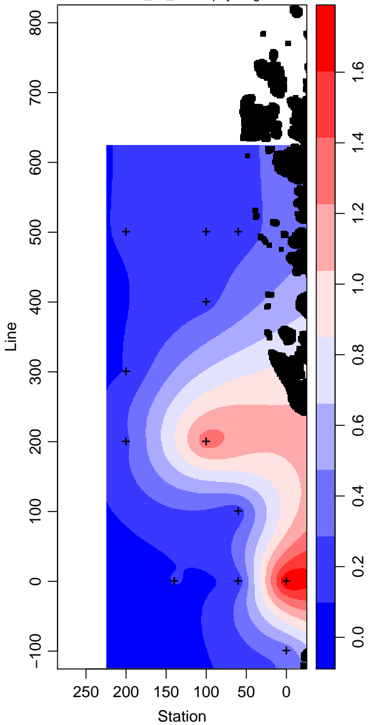
LMG13-01_80_Chlorophyll mg m -3
