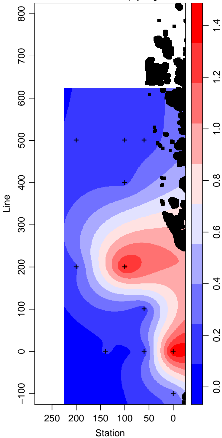
LMG13-01_85_Chlorophyll mg m -3
