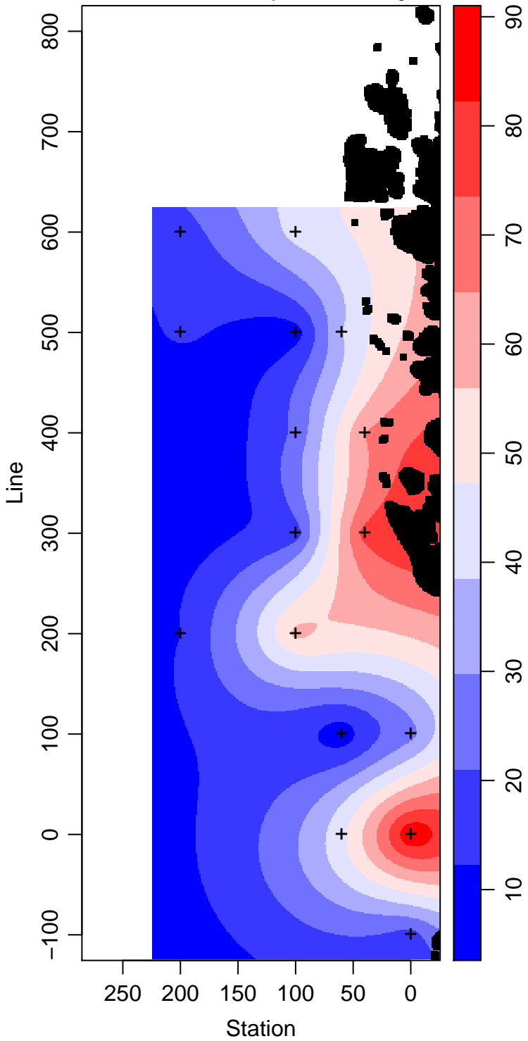
LMG13-01_25_Primary.Production mg m -3
