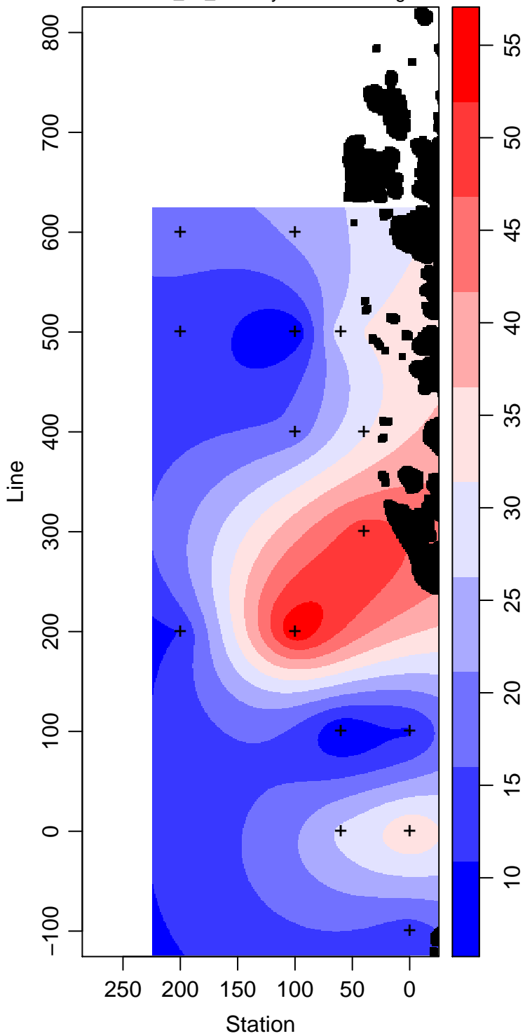
LMG13-01_35_Primary.Production mg m -3
