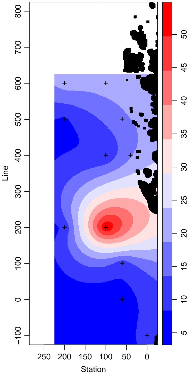
LMG13-01_50_Primary.Production mg m -3
