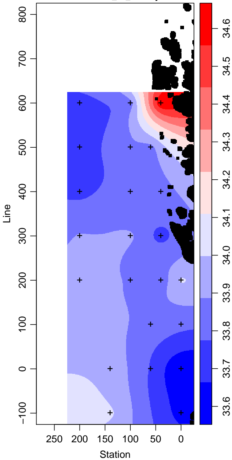
LMG13-01_35_Salinity
