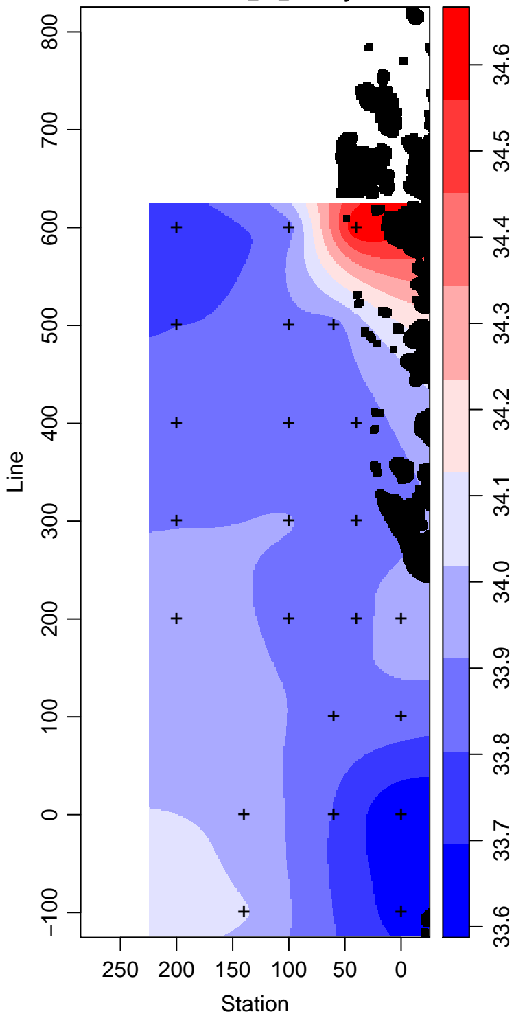
LMG13-01_40_Salinity
