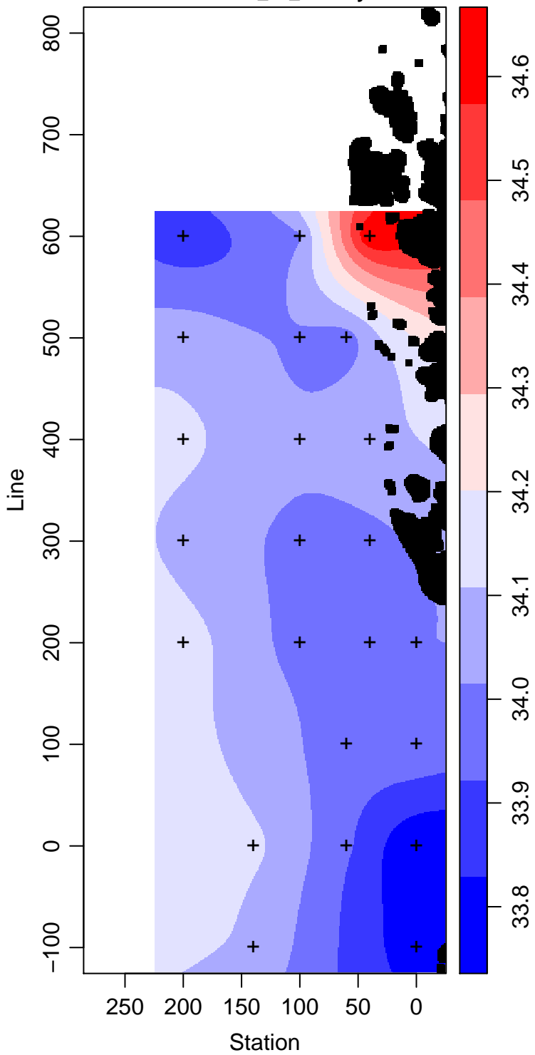
LMG13-01_75_Salinity
