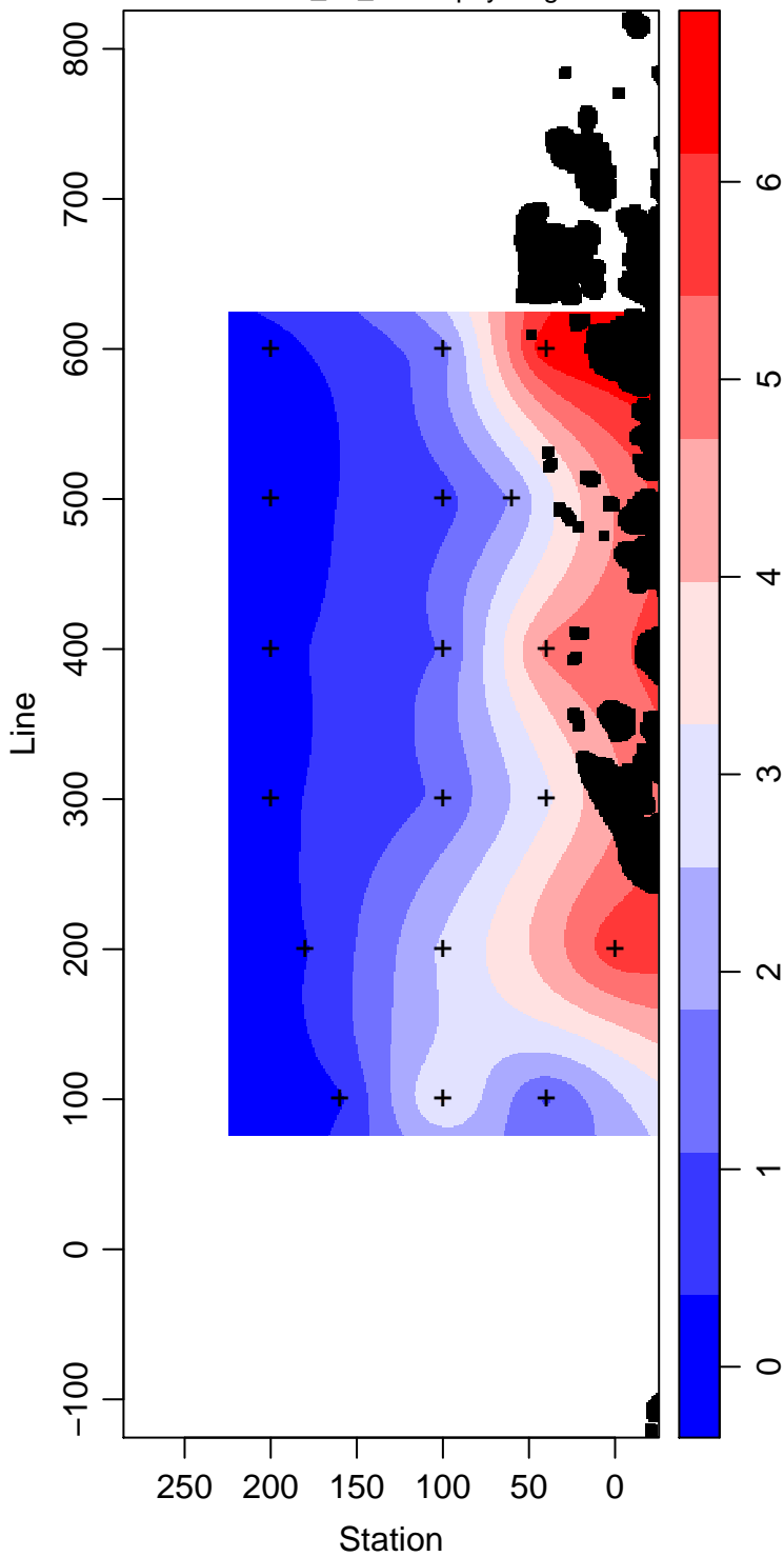
LMG14-01_20_Chlorophyll mg m -3
