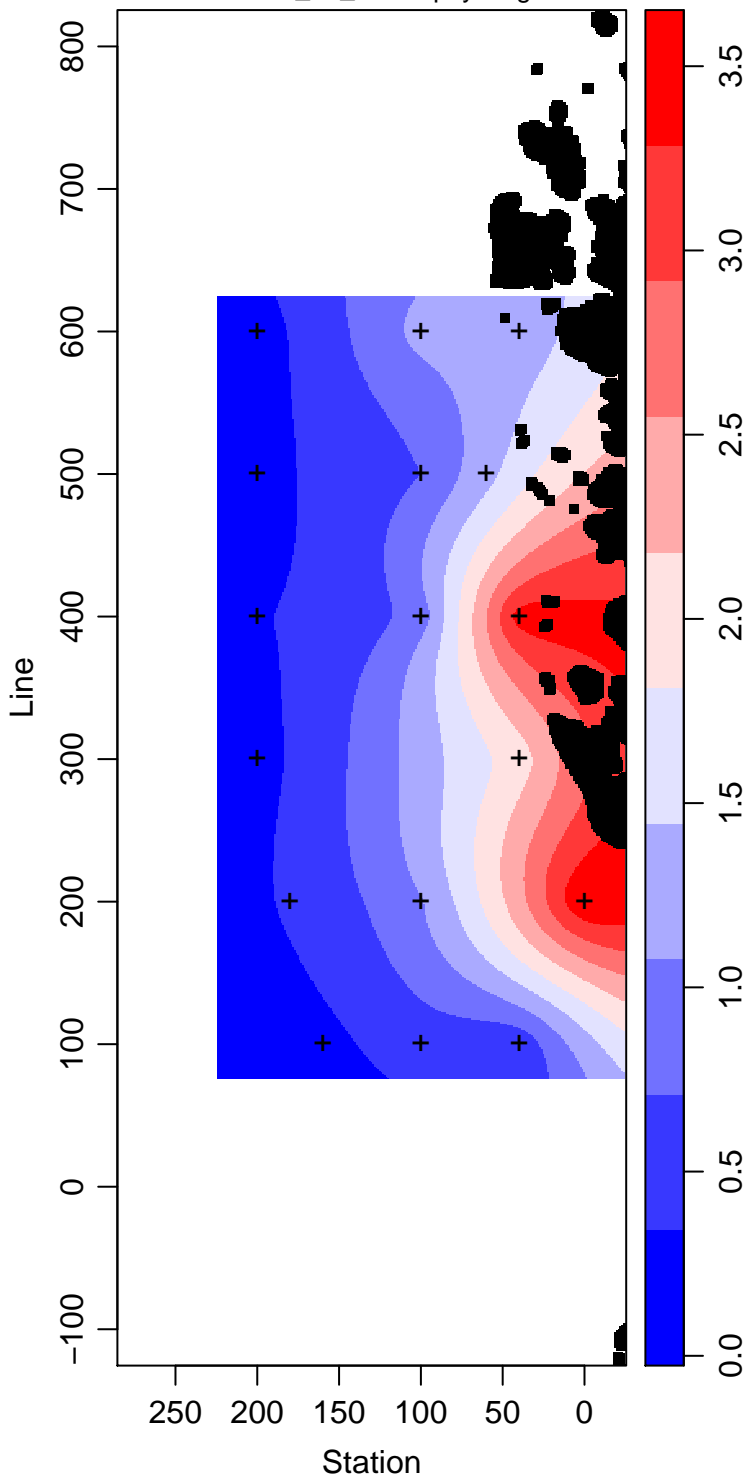
LMG14-01_30_Chlorophyll mg m -3
