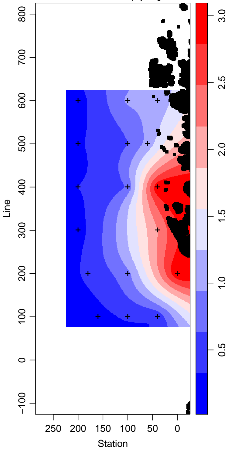
LMG14-01_35_Chlorophyll mg m -3
