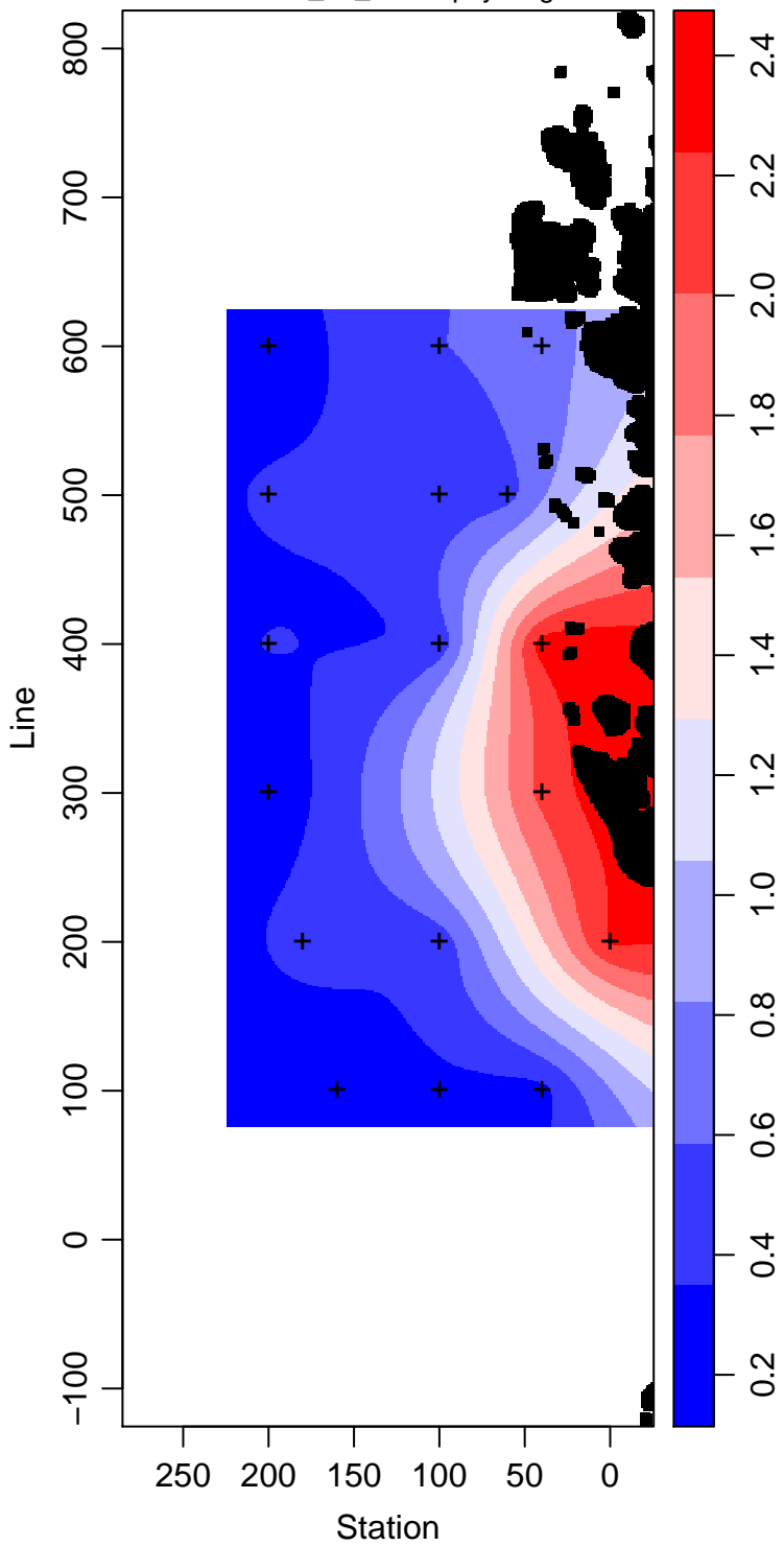
LMG14-01_45_Chlorophyll mg m -3
