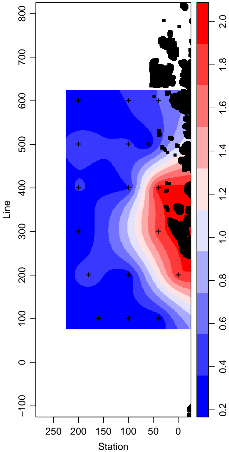
LMG14-01_50_Chlorophyll mg m -3
