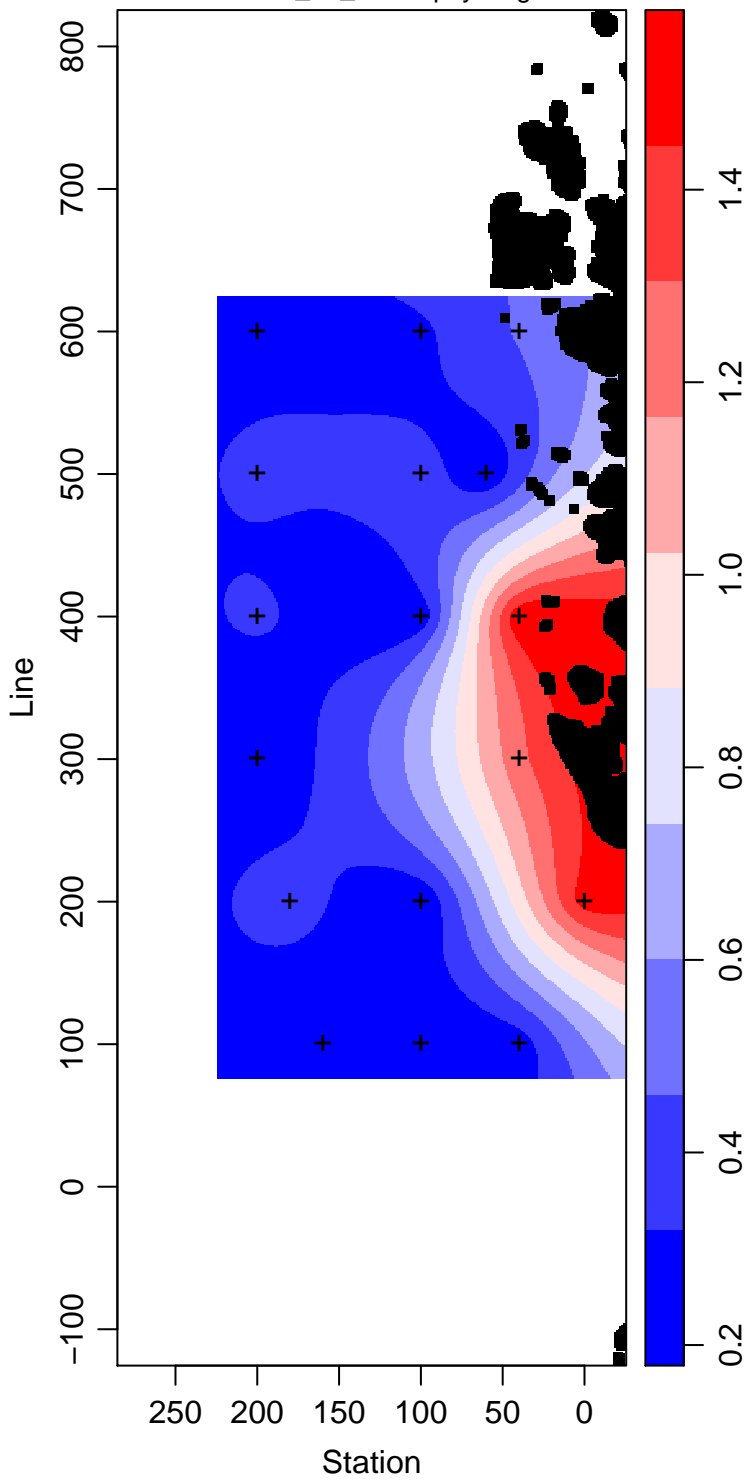
LMG14-01_60_Chlorophyll mg m -3
