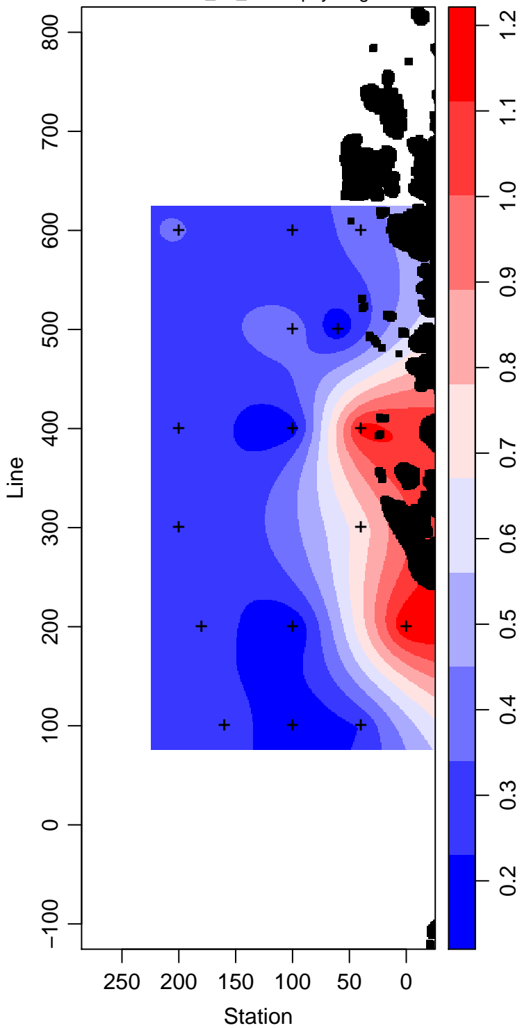
LMG14-01_70_Chlorophyll mg m -3
