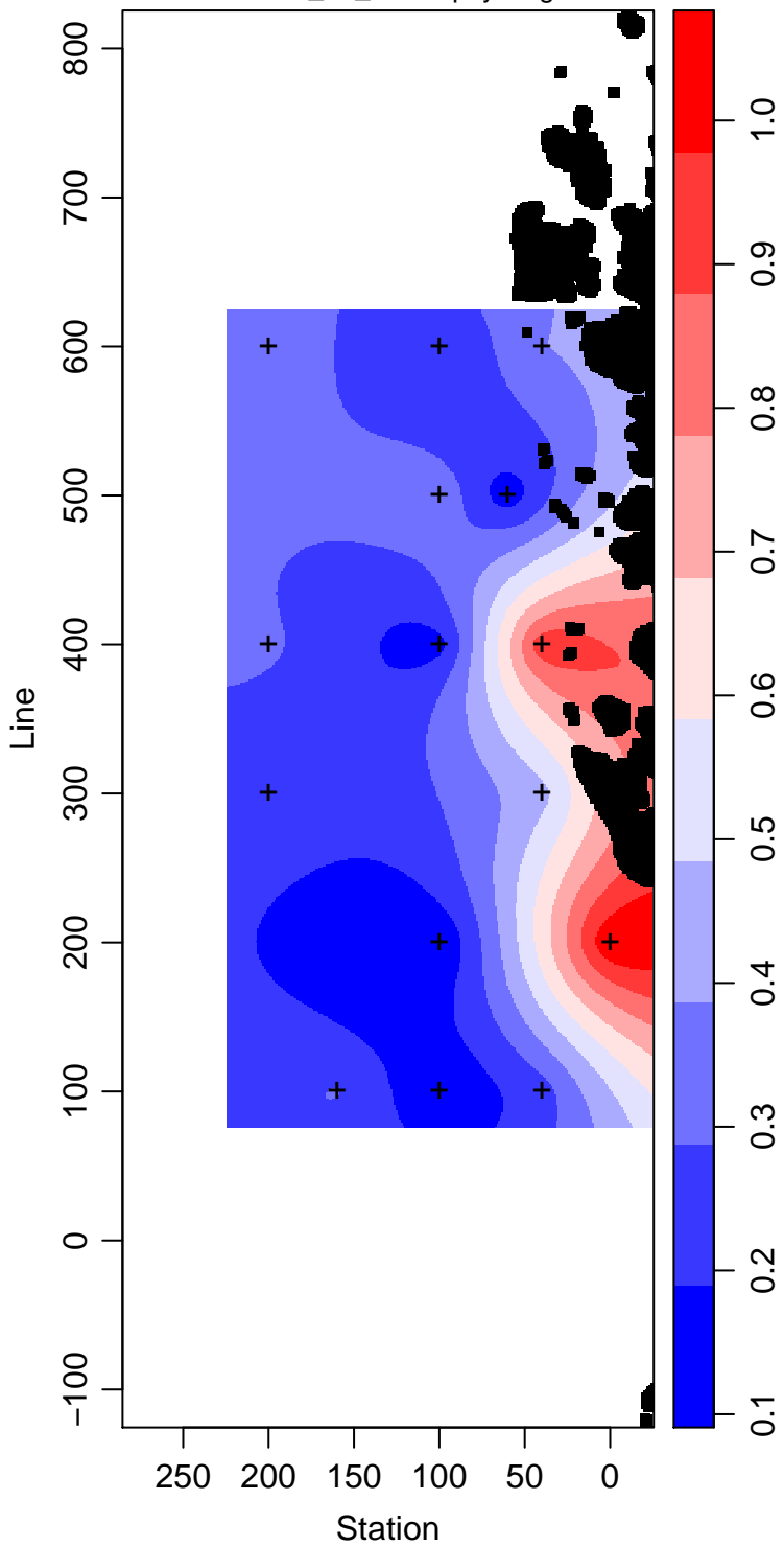
LMG14-01_75_Chlorophyll mg m -3
