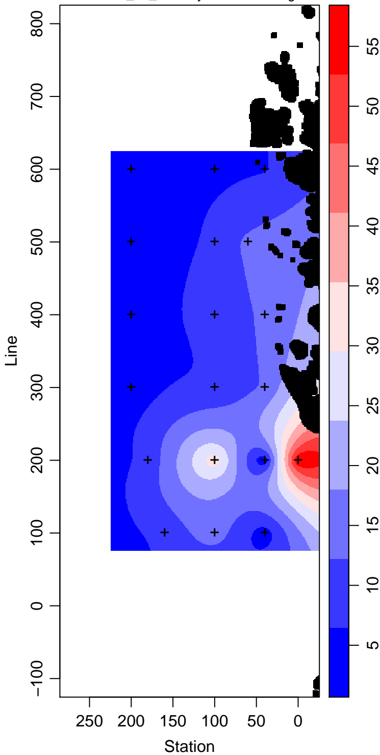
LMG14-01_35_Primary.Production mg m -3
