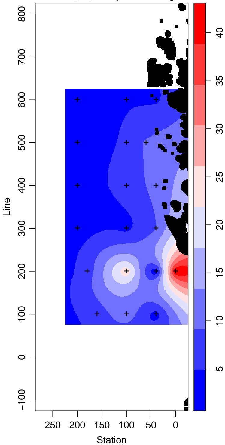
LMG14-01_40_Primary.Production mg m -3
