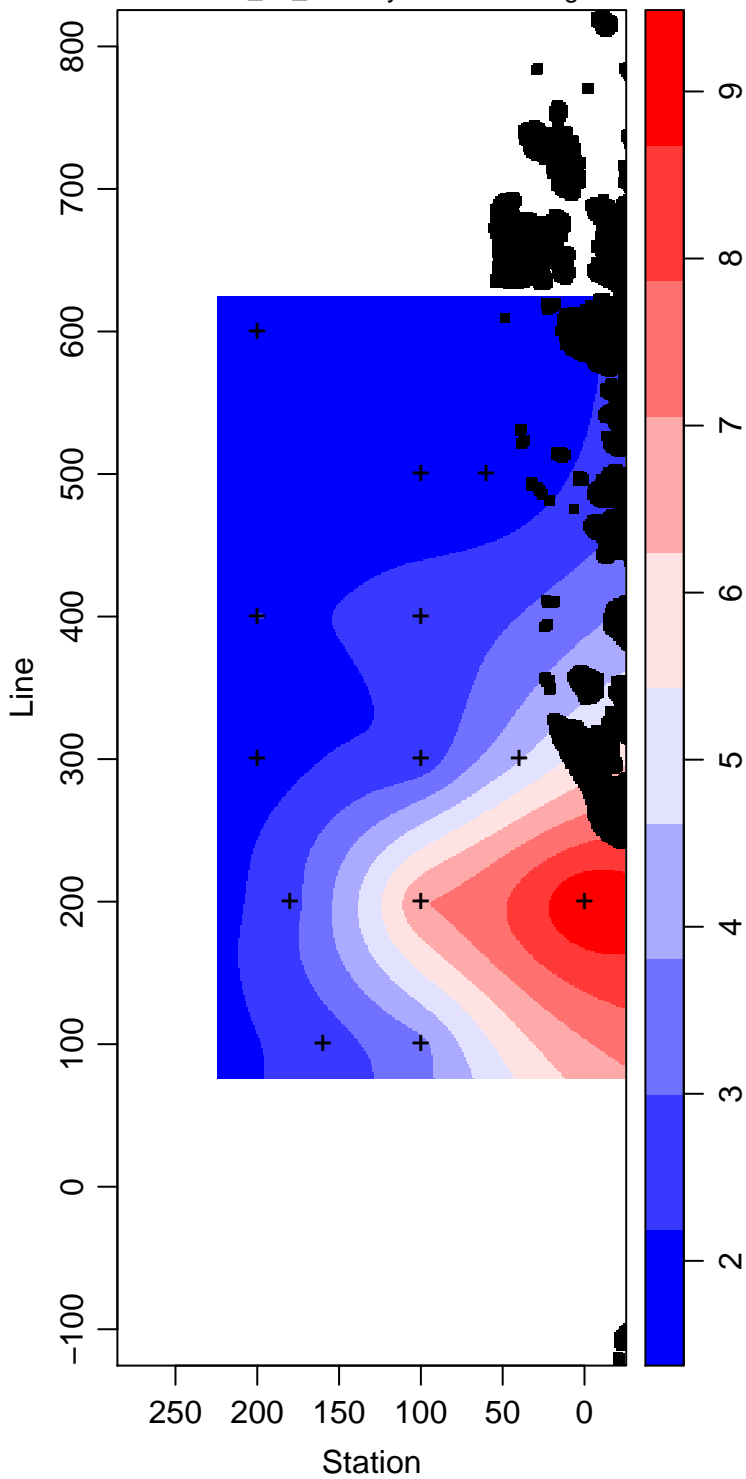
LMG14-01_60_Primary.Production mg m -3
