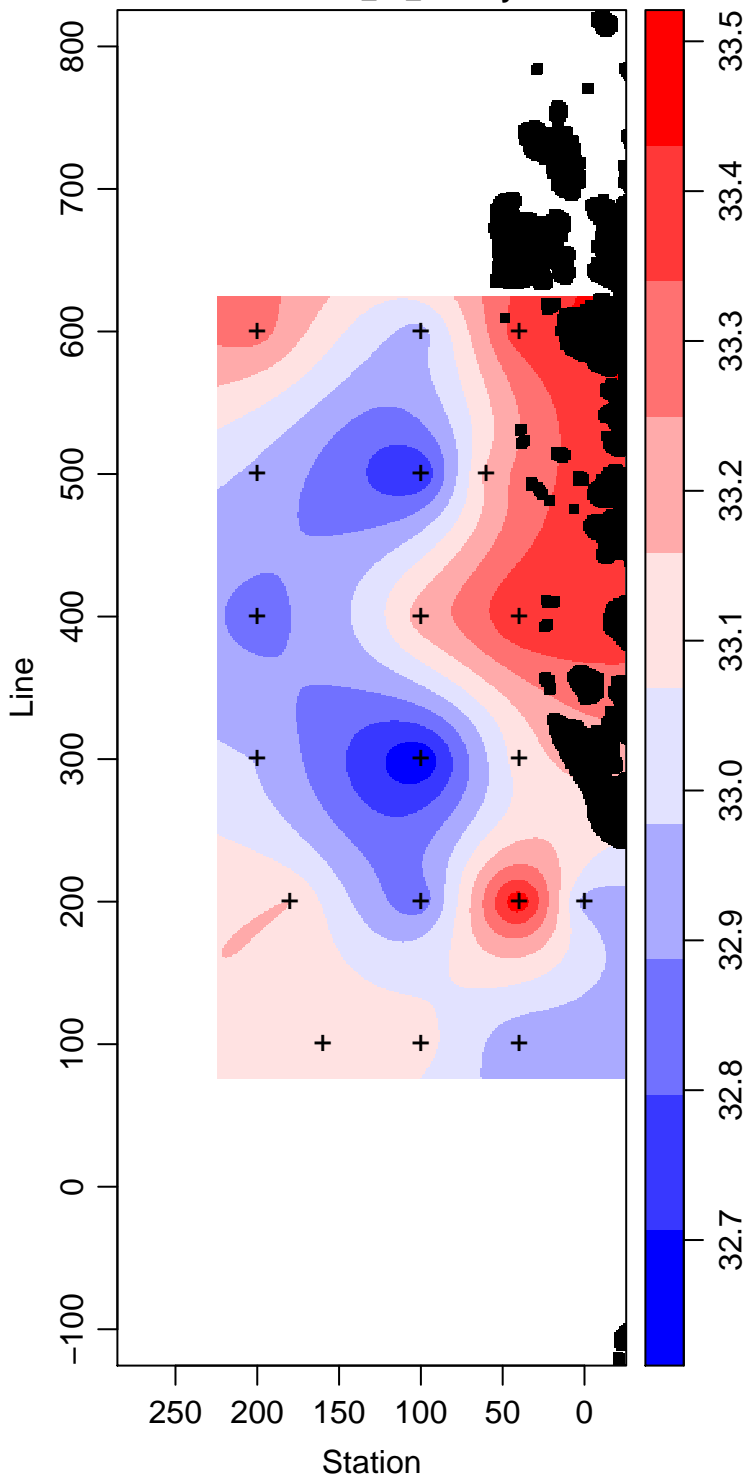
LMG14-01_10_Salinity
