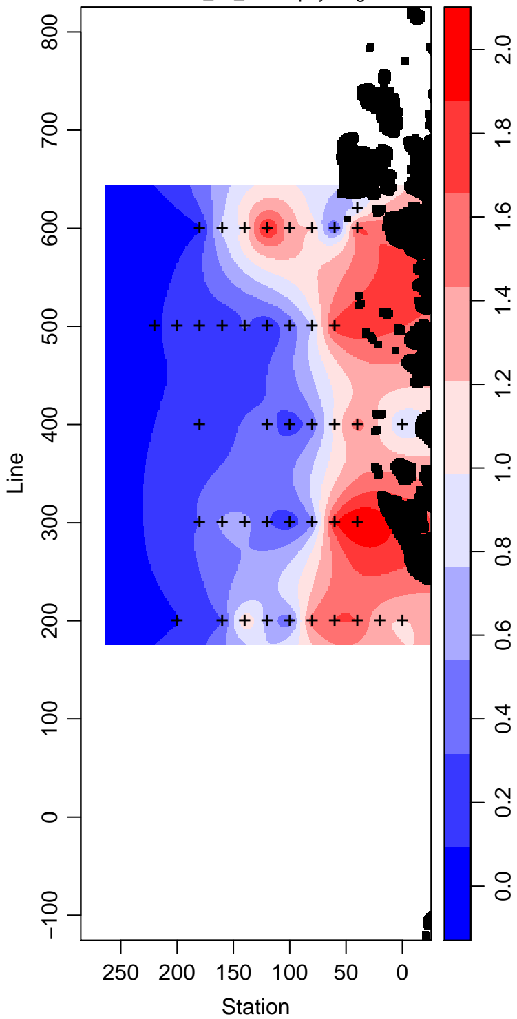
LMG99-01_10_Chlorophyll mg m -3
