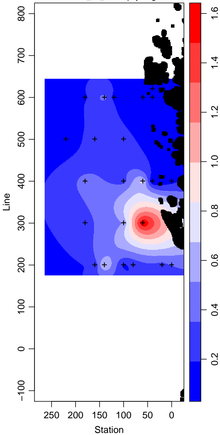
LMG99-01_50_Chlorophyll mg m -3
