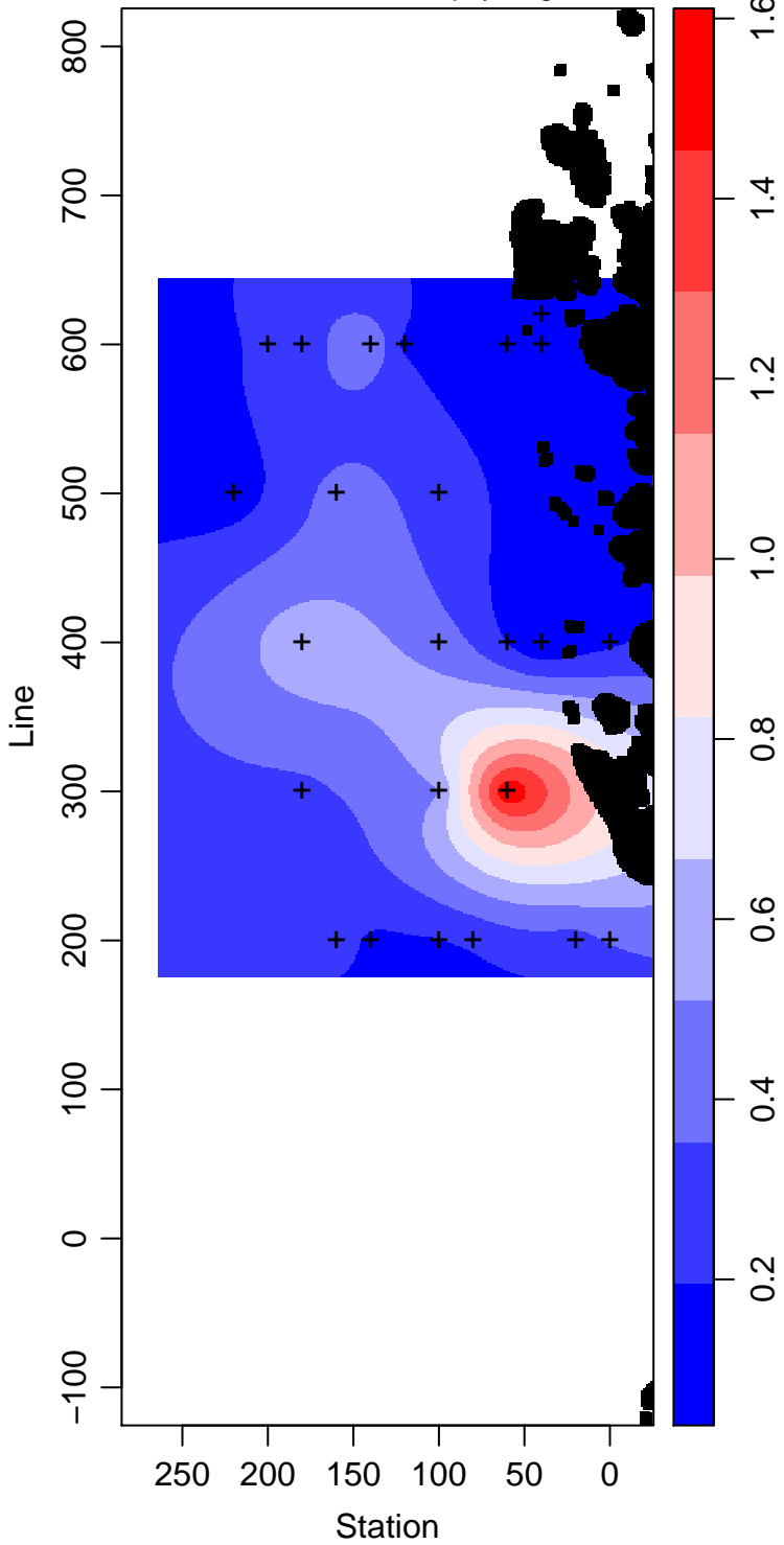
LMG99-01_55_Chlorophyll mg m -3
