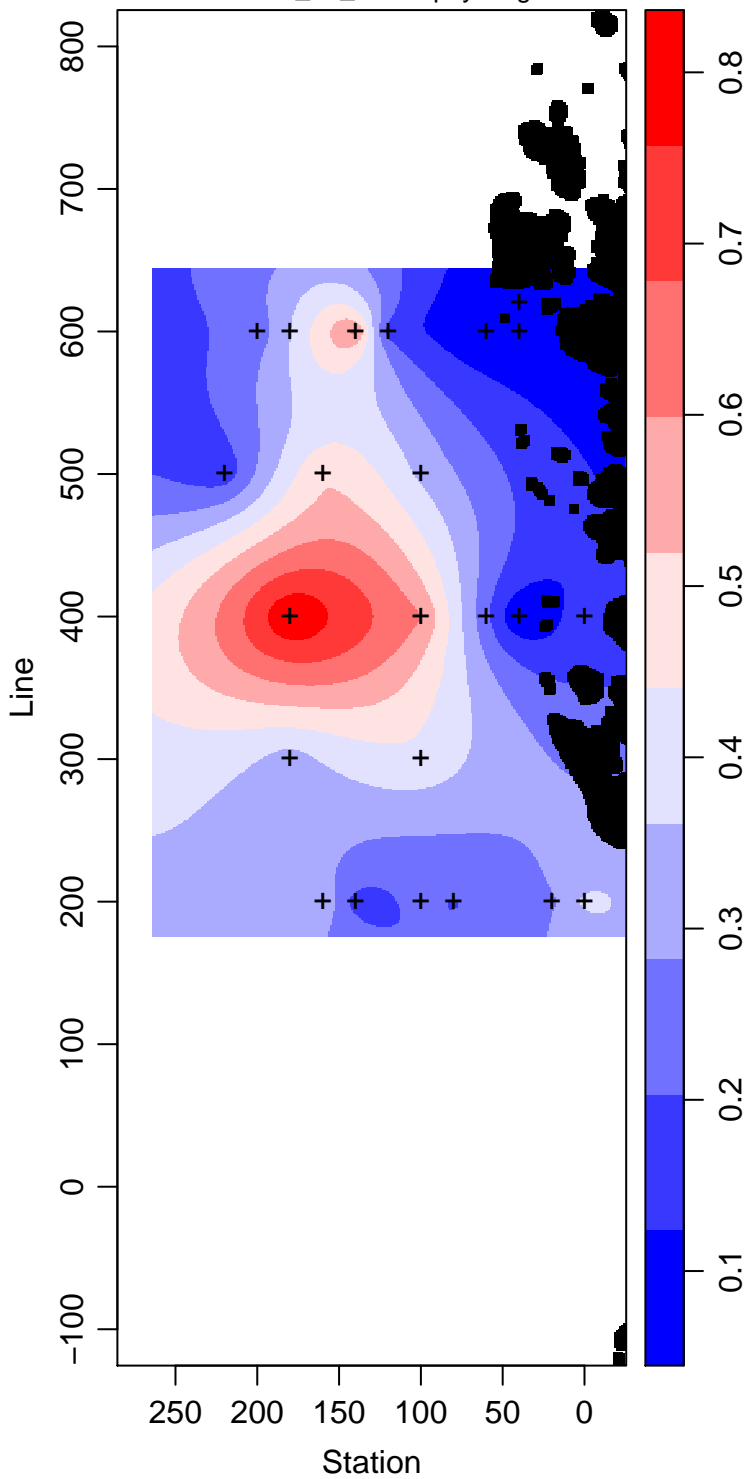
LMG99-01_60_Chlorophyll mg m -3
