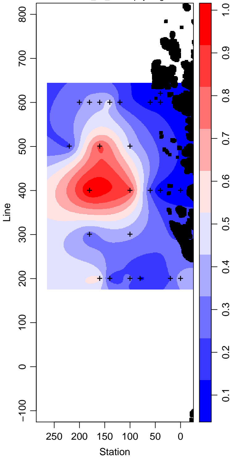
LMG99-01_75_Chlorophyll mg m -3
