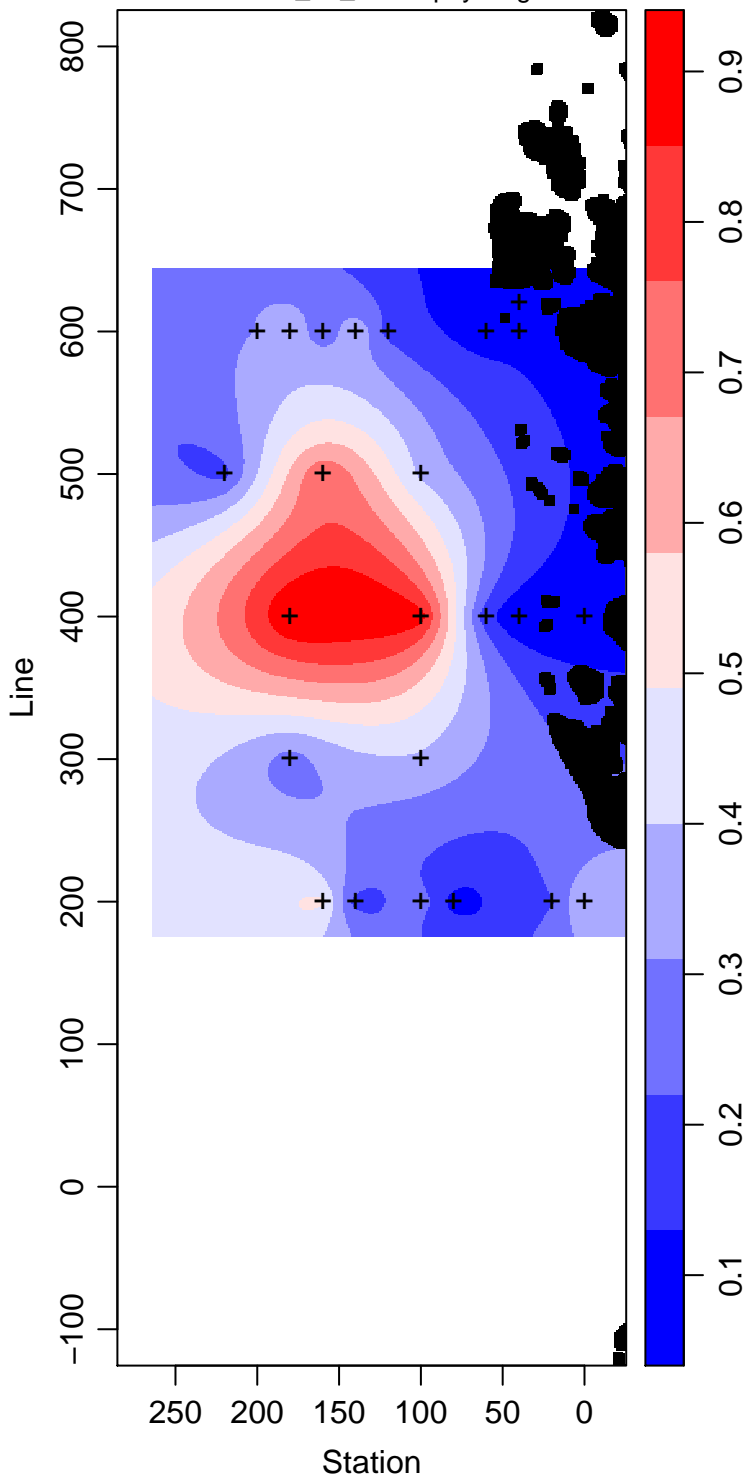
LMG99-01_80_Chlorophyll \text{mg m}^{-3}
