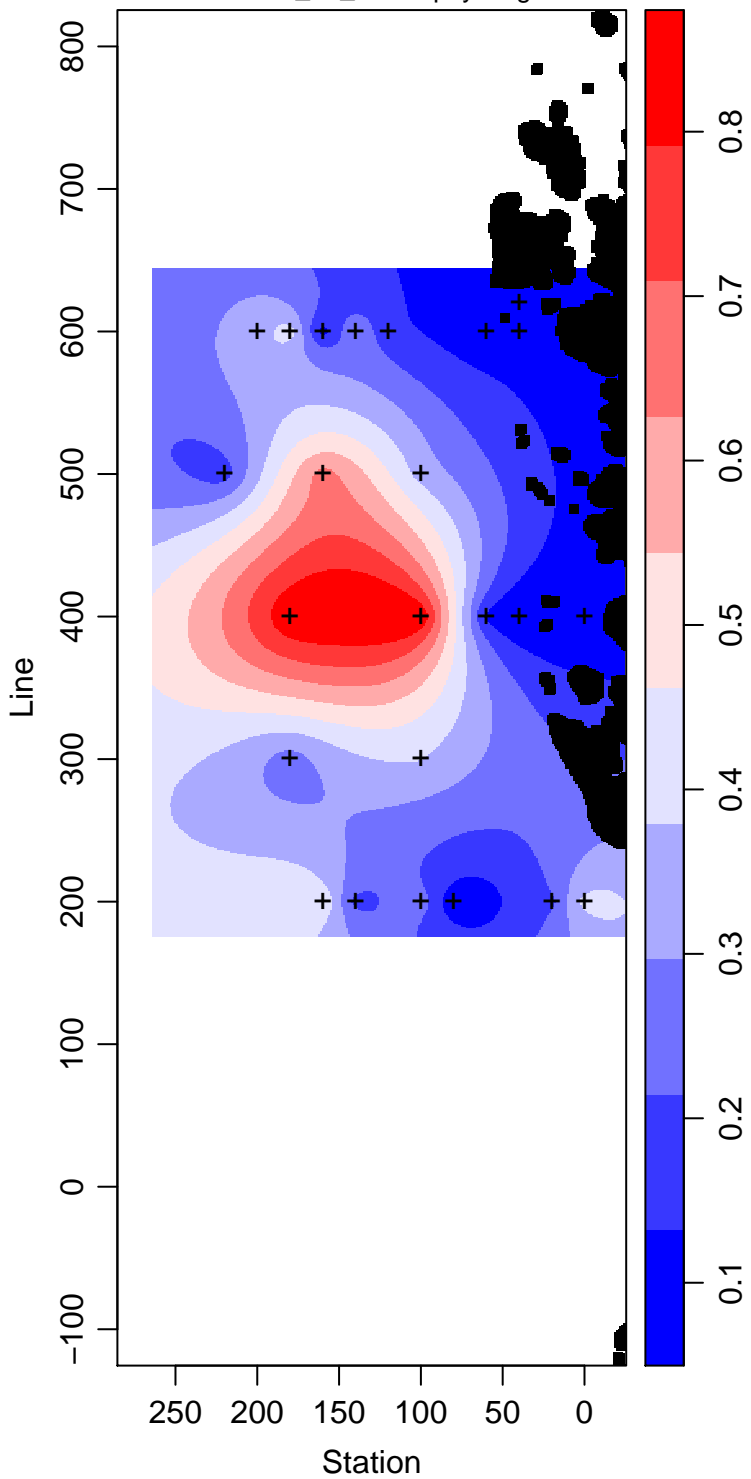
LMG99-01_85_Chlorophyll mg m -3
