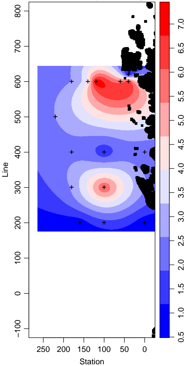
LMG99-01_35_Primary.Production mg m -3
