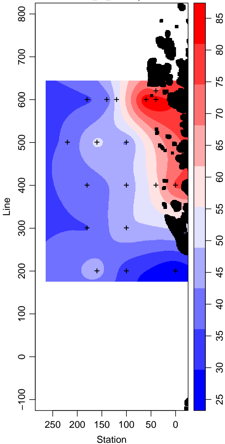
LMG99-01_35_Silicate \mu\text{ mol L}^{-1}
