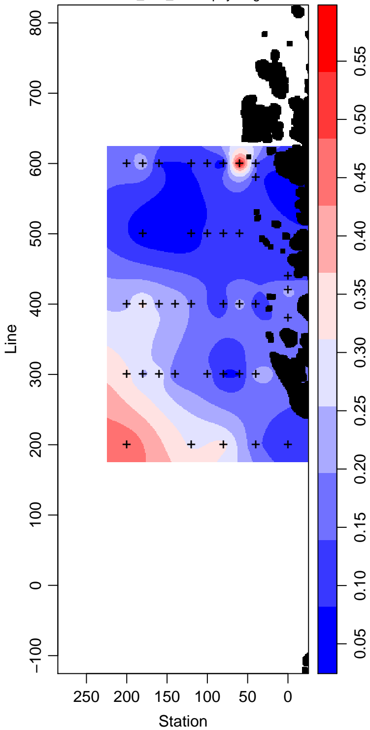
PD93-01_100_Chlorophyll mg m -3
