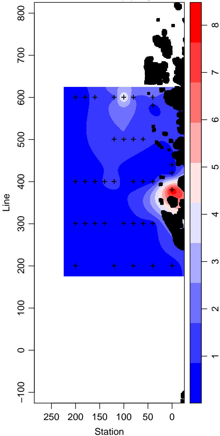
PD93-01_1_Chlorophyll \text{mg m}^{-3}
