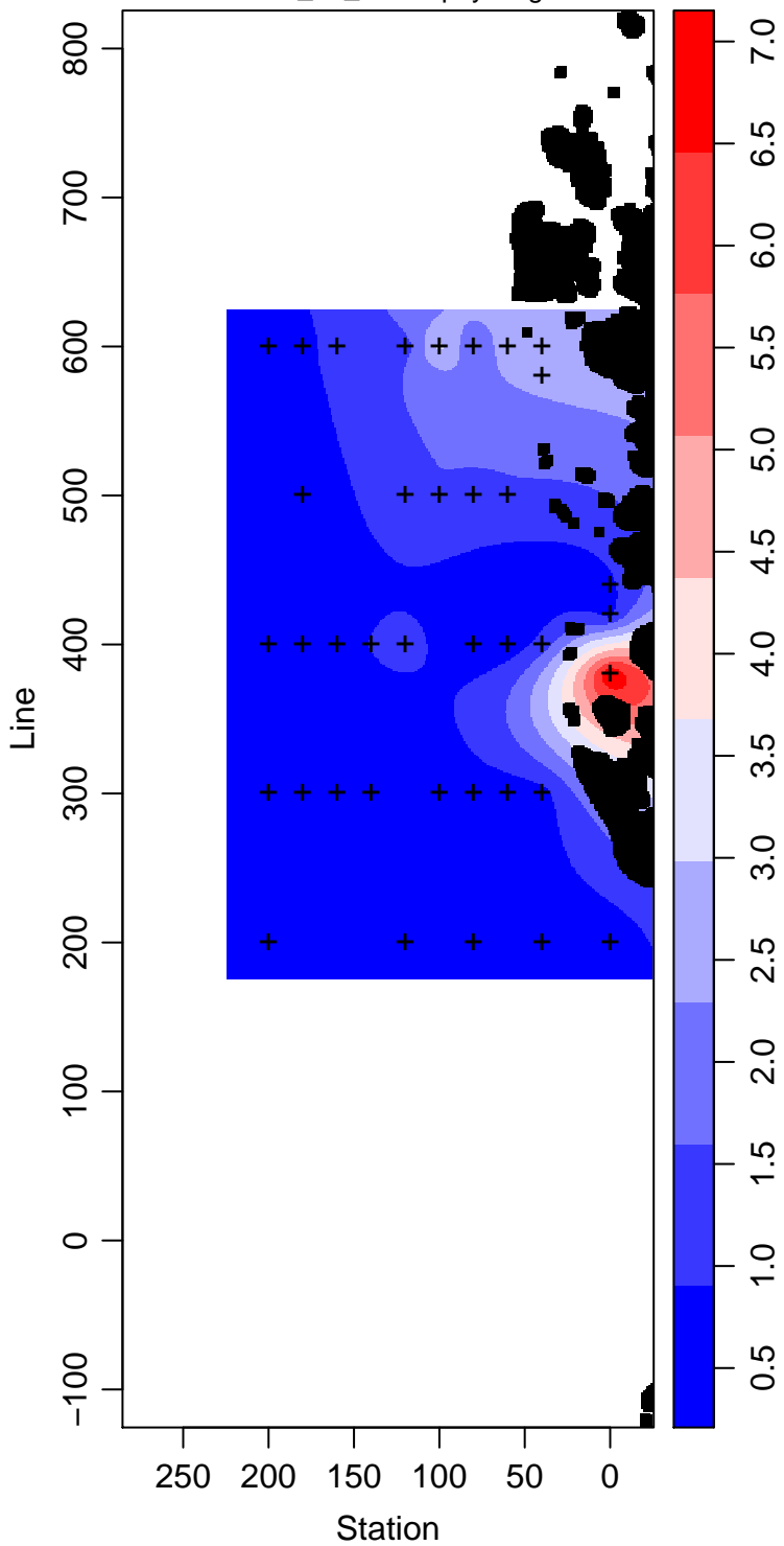
PD93-01_20_Chlorophyll mg m -3
