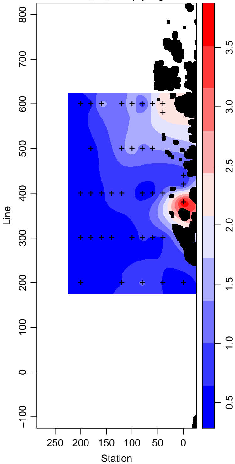
PD93-01_25_Chlorophyll mg m -3
