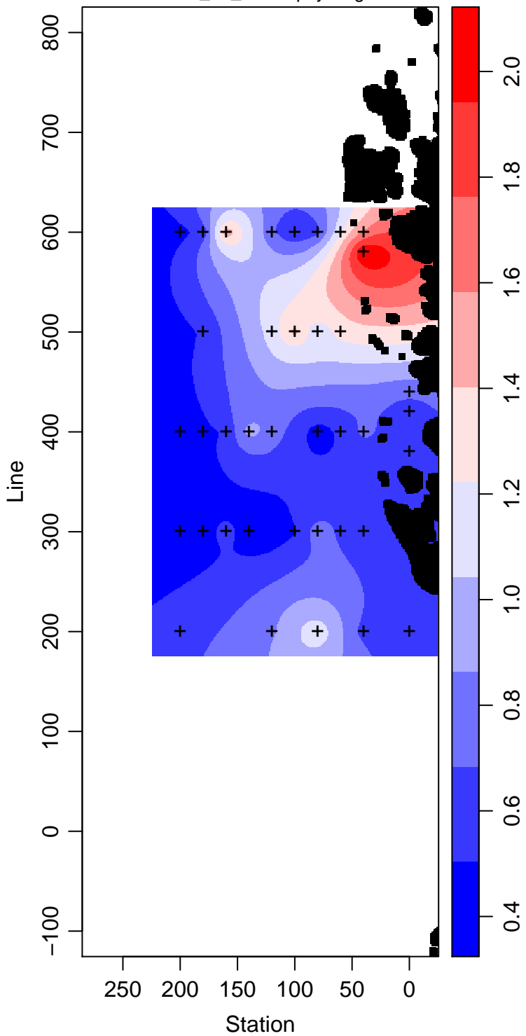
PD93-01_30_Chlorophyll mg m -3
