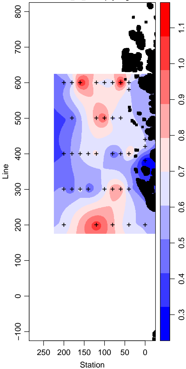
PD93-01_40_Chlorophyll mg m -3
