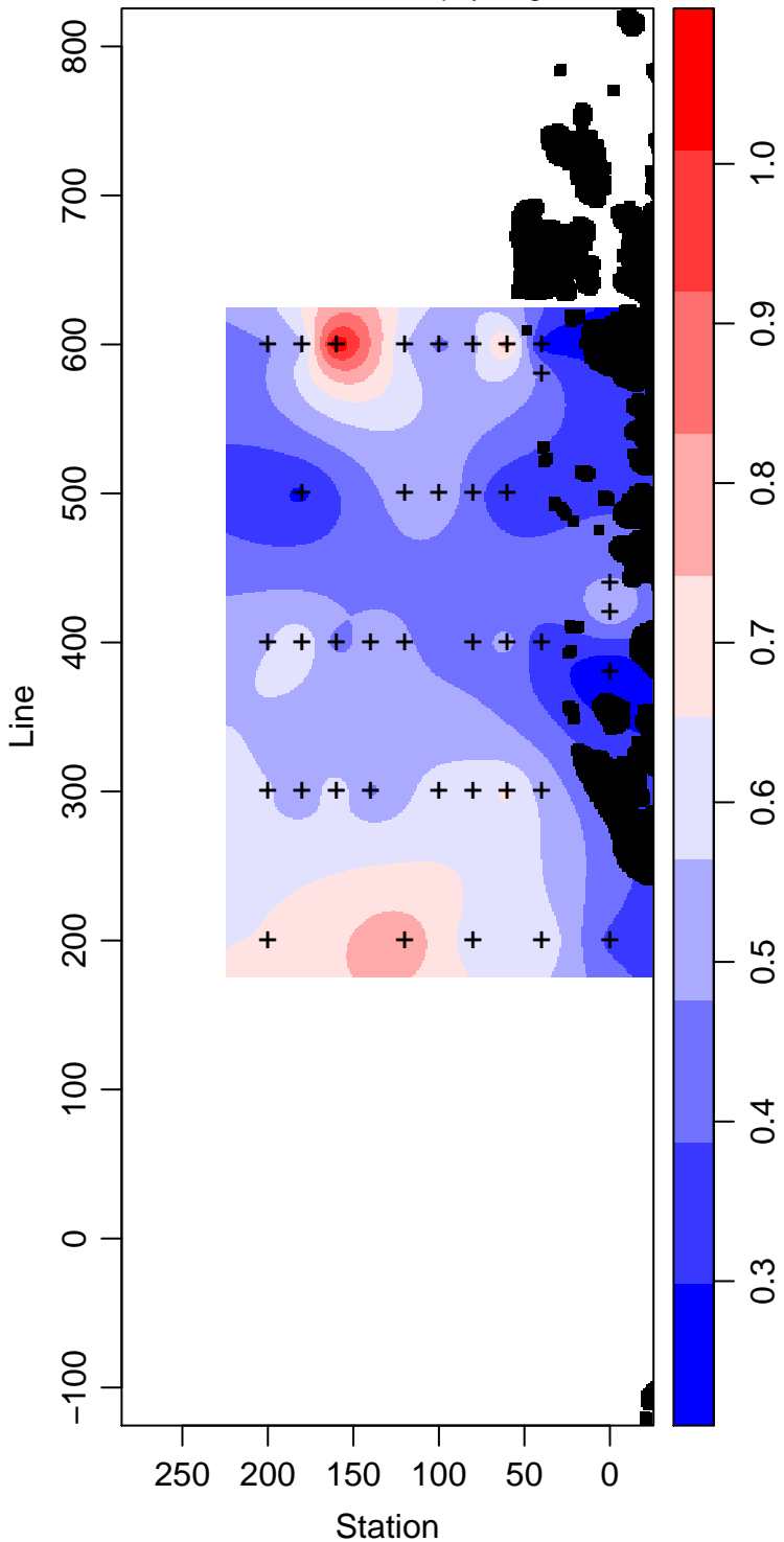
PD93-01_60_Chlorophyll mg m -3
