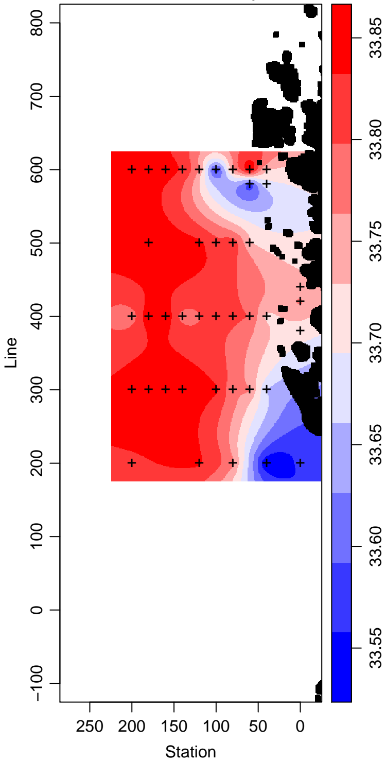
PD93-01_40_Salinity
