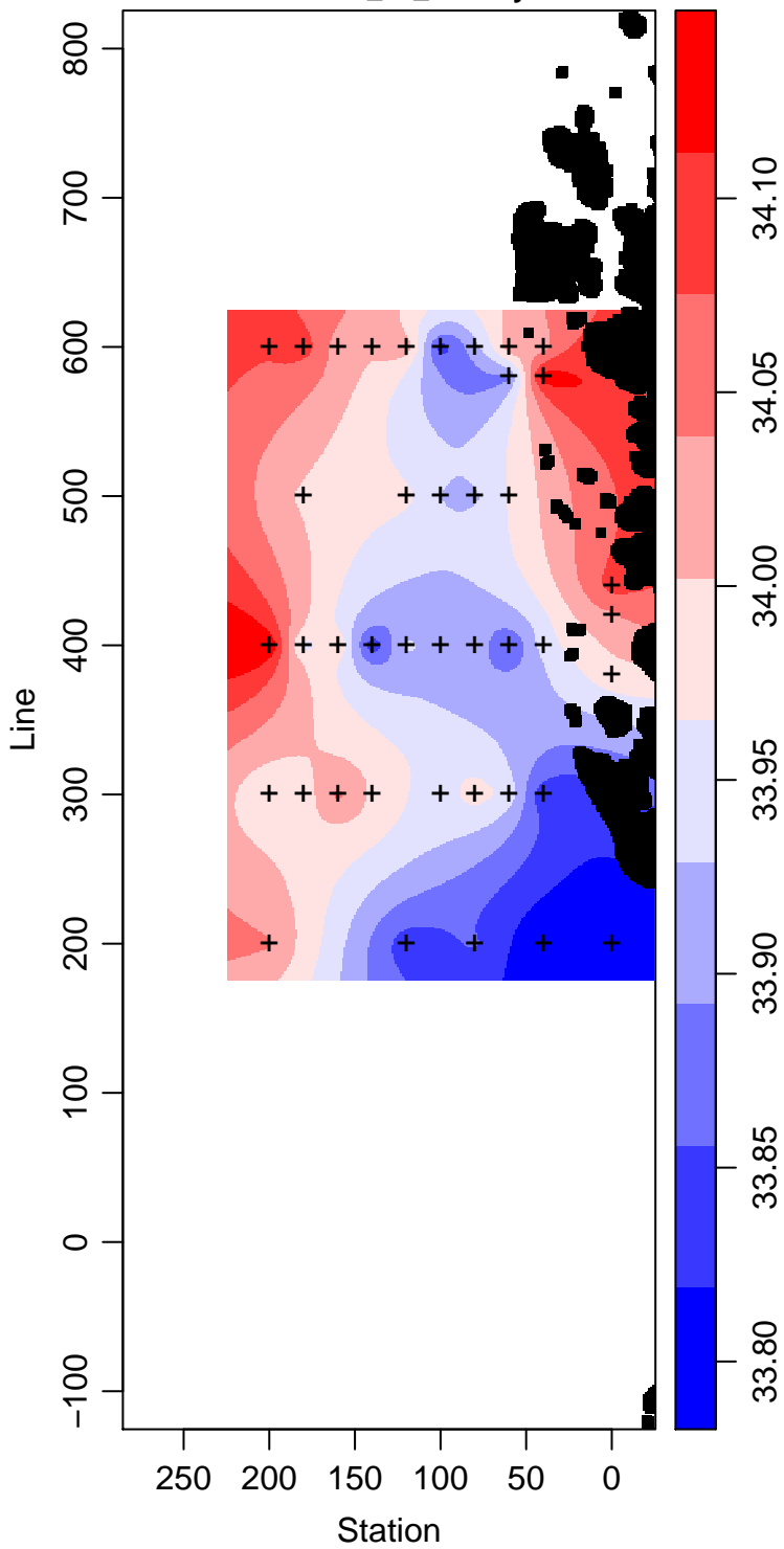
PD93-01_90_Salinity
