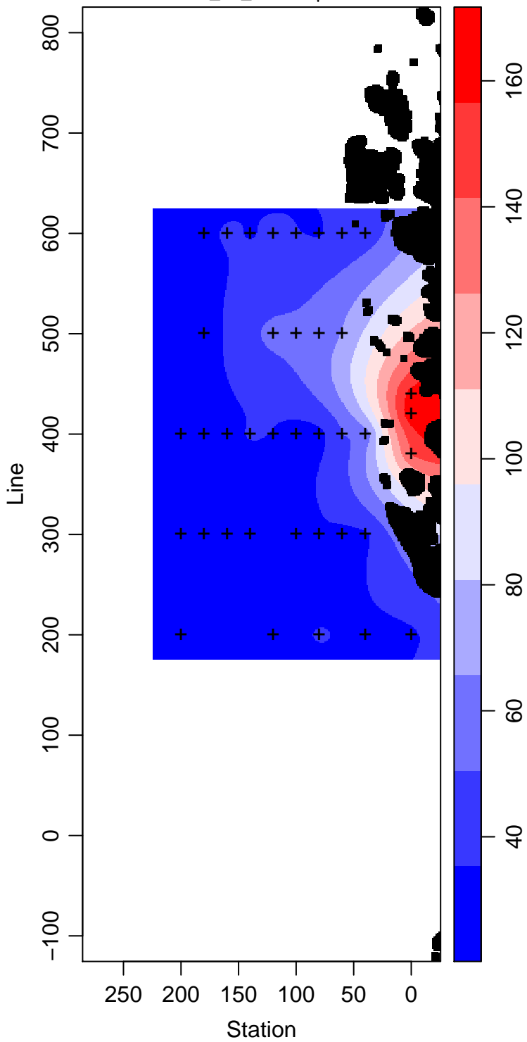
PD93-01_35_Silicate \mu\text{ mol L}^{-1}
