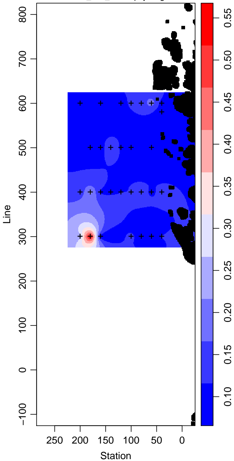
PD94-01_100_Chlorophyll mg m -3
