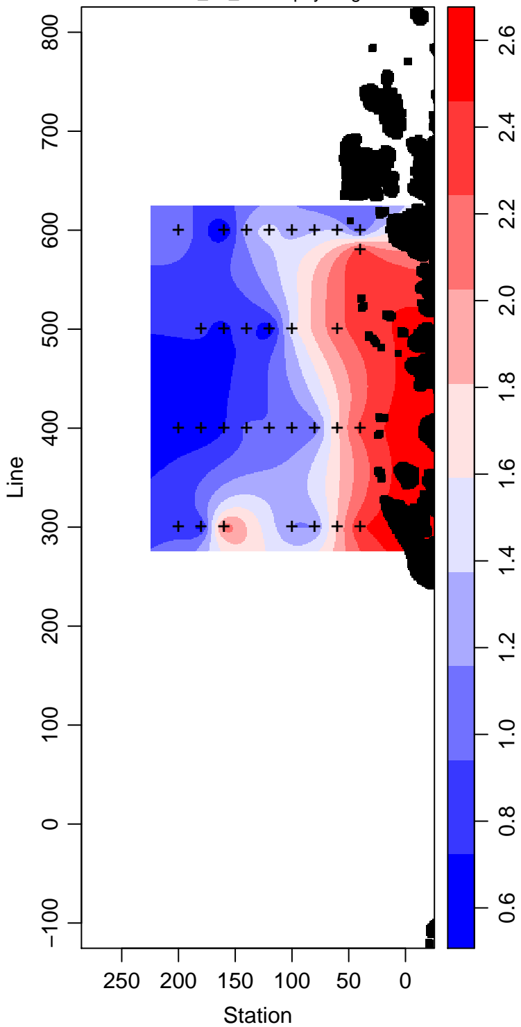
PD94-01_15_Chlorophyll \text{mg m}^{-3}
