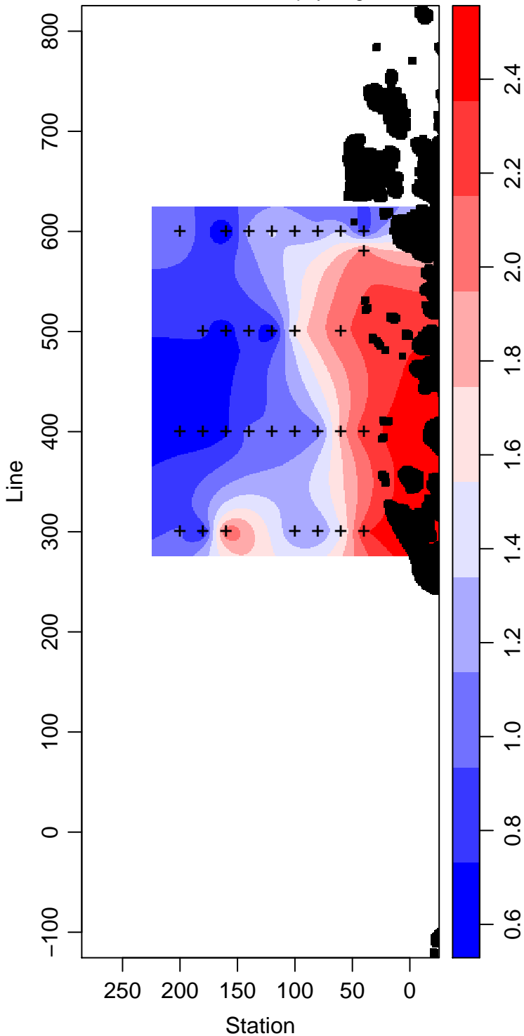
PD94-01_20_Chlorophyll mg m -3
