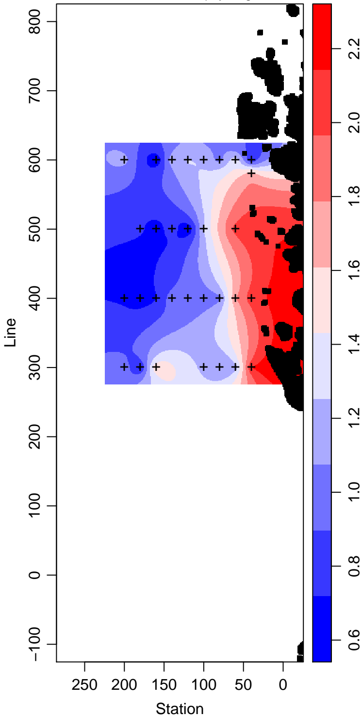
PD94-01_25_Chlorophyll mg m -3
