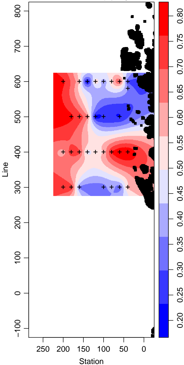
PD94-01_55_Chlorophyll mg m -3
