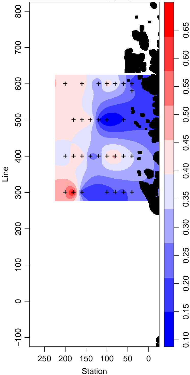
PD94-01_70_Chlorophyll mg m -3
