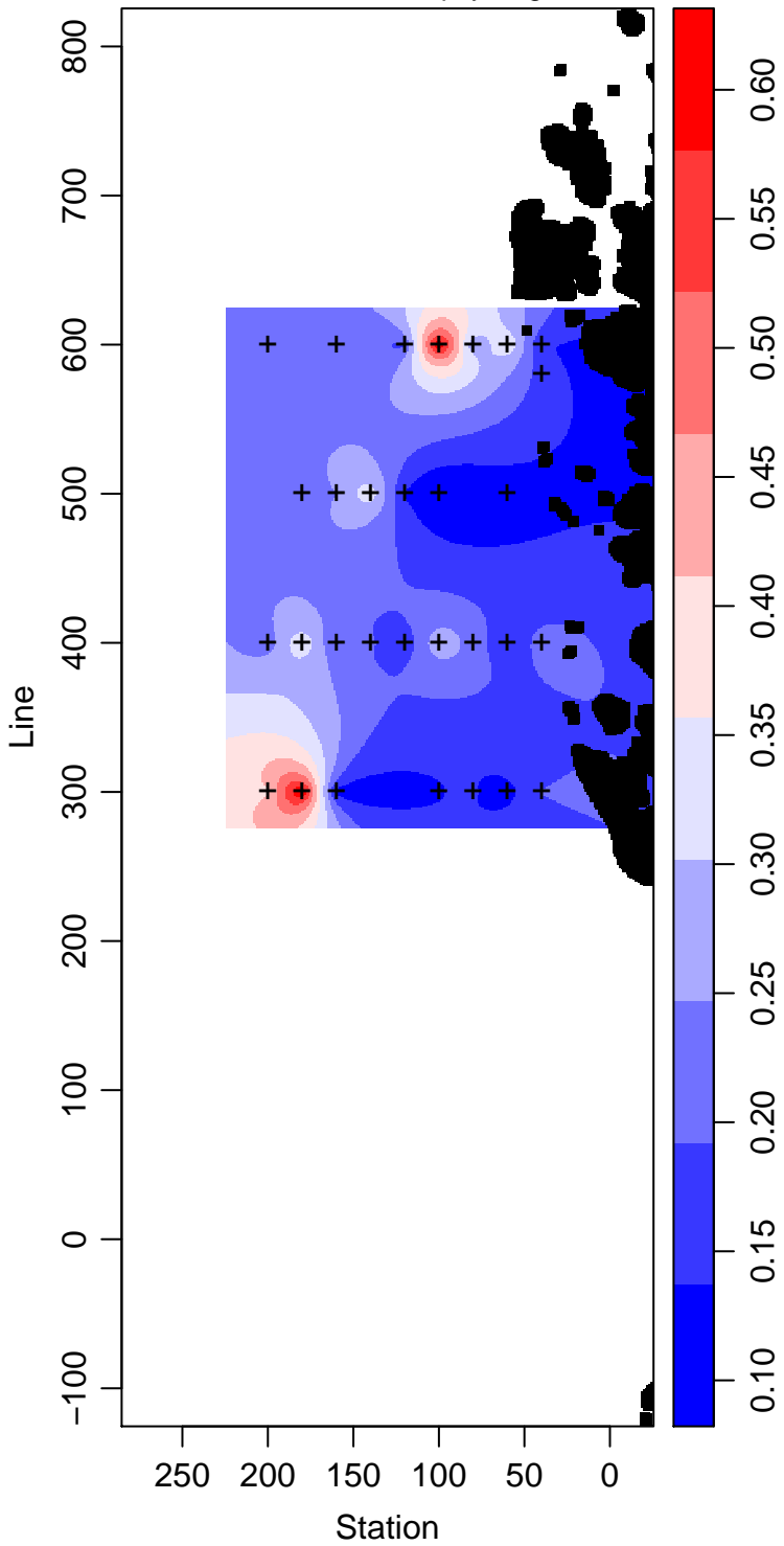
PD94-01_80_Chlorophyll mg m -3
